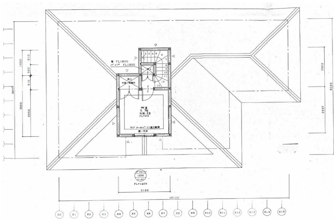
2階平面図
