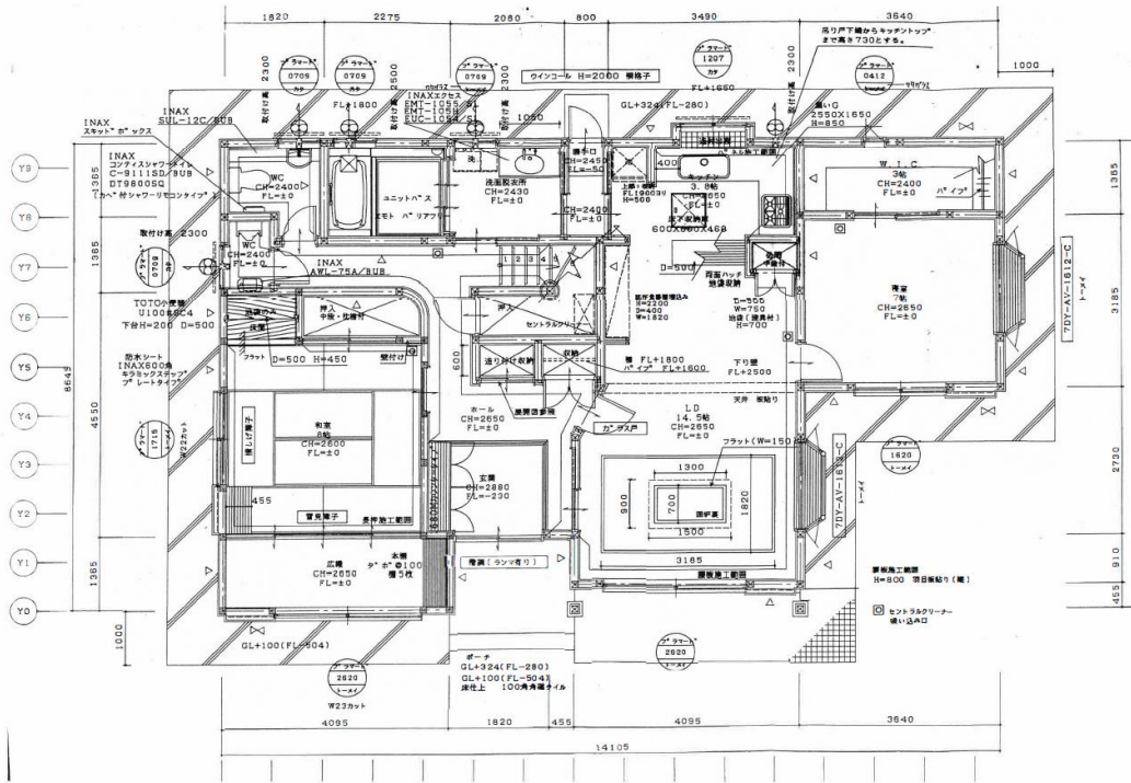
1階平面図
