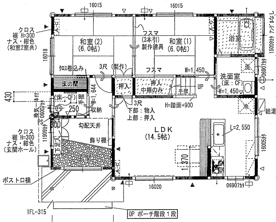
1階平面図
